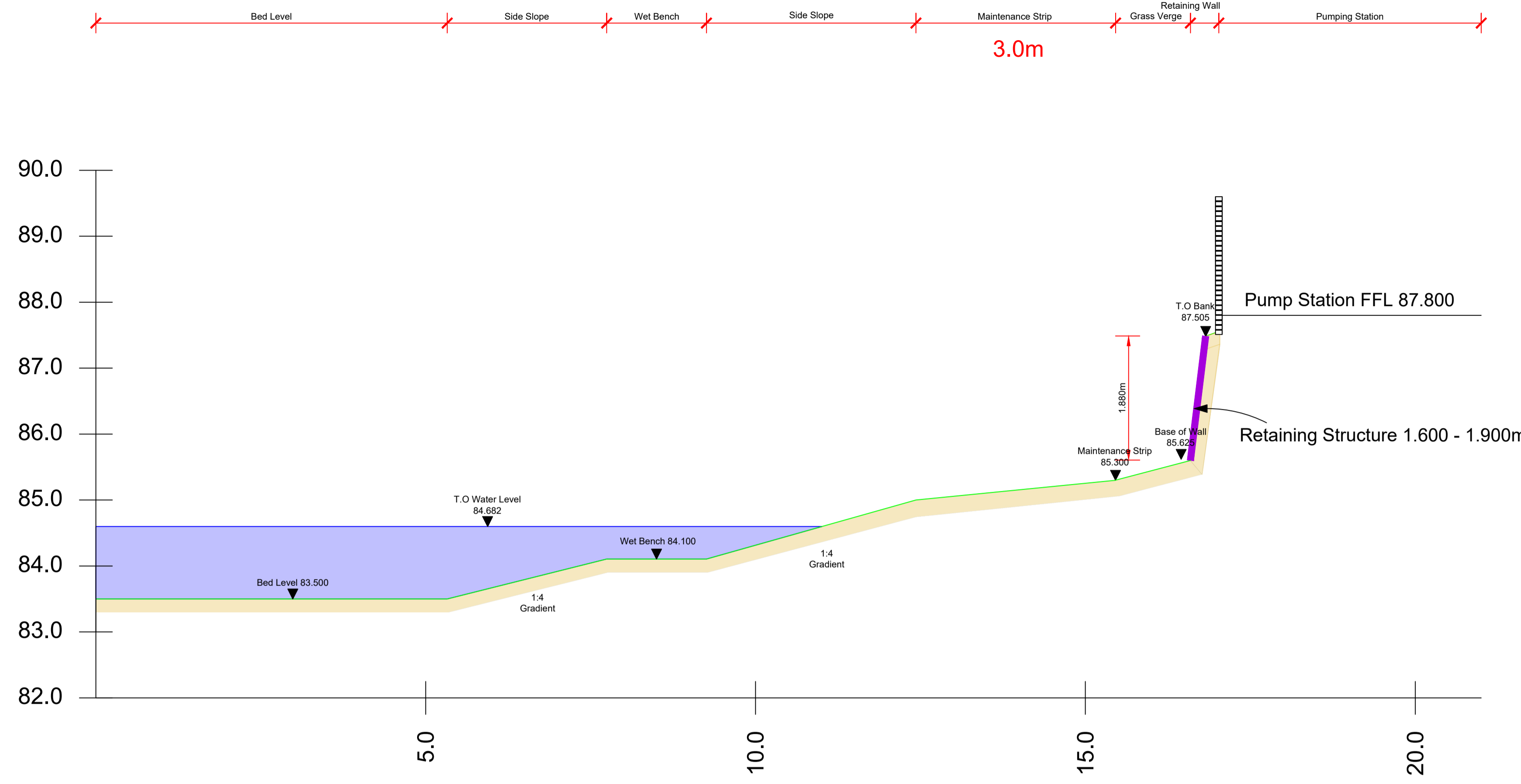
SECTION A-A
